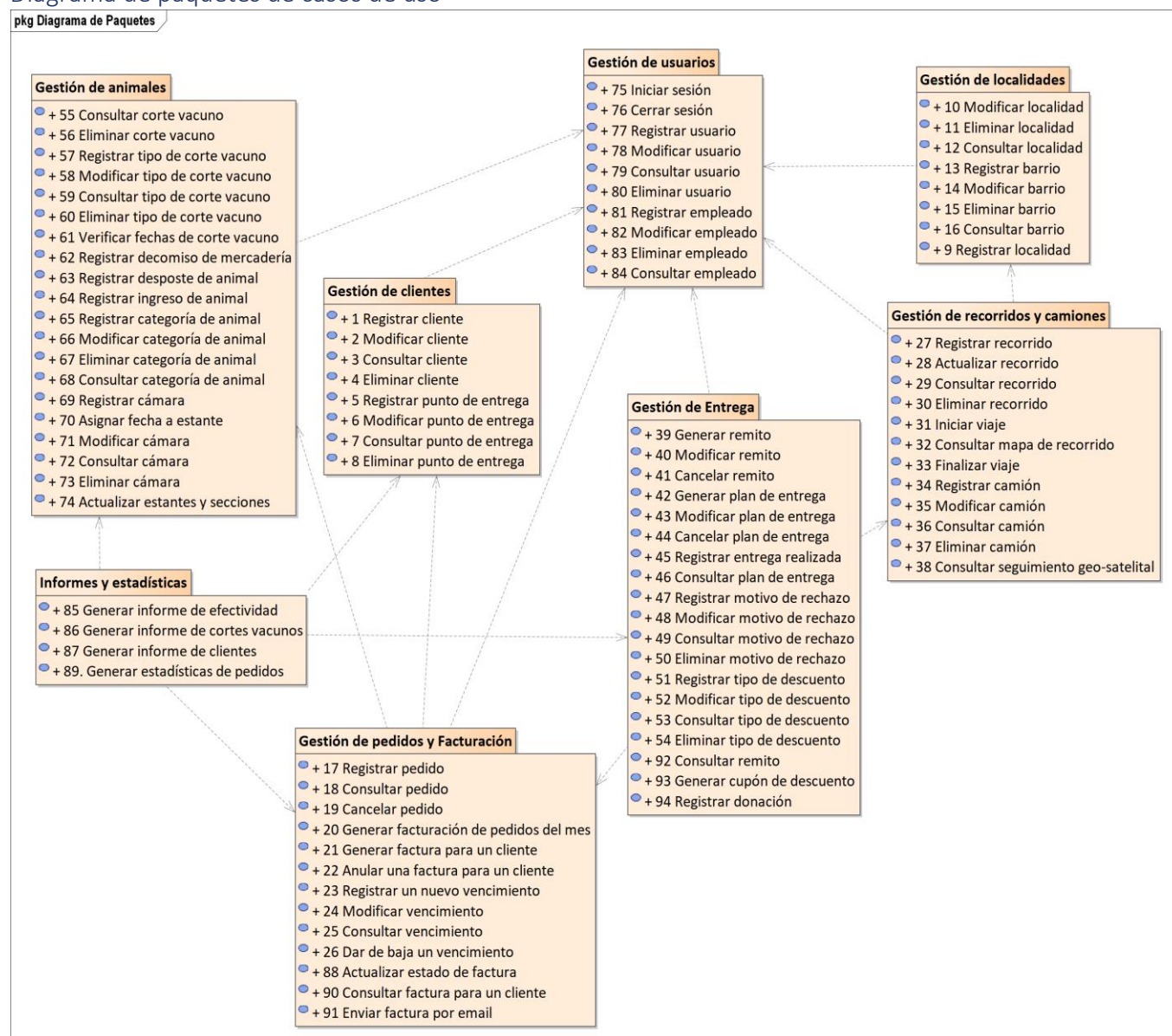
Diagrama de paquetes de casos de uso
